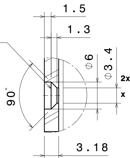
DETALLE B ESCALA: 2:1
